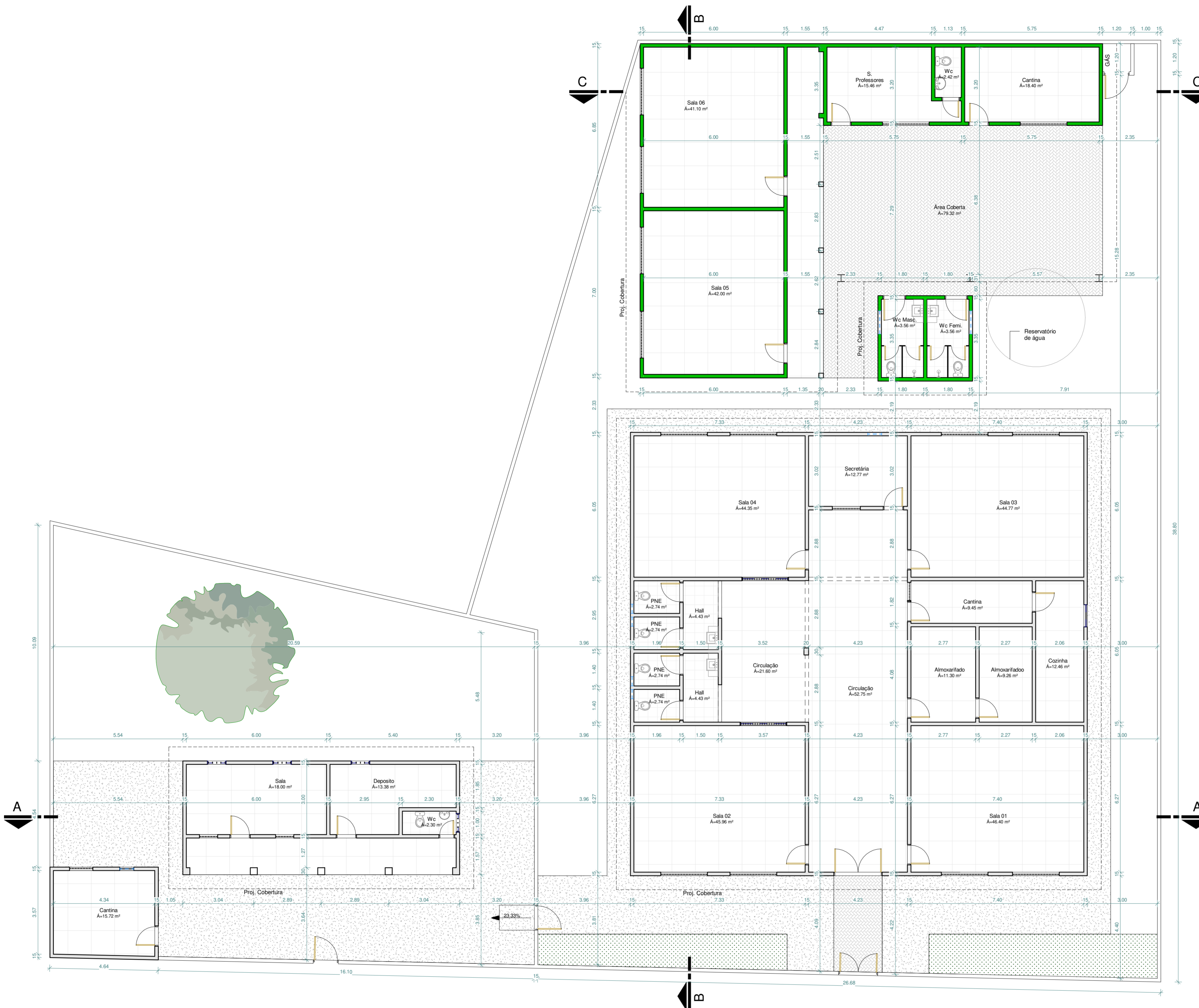
1 PLANTA DE REFORMA 1 : 100
