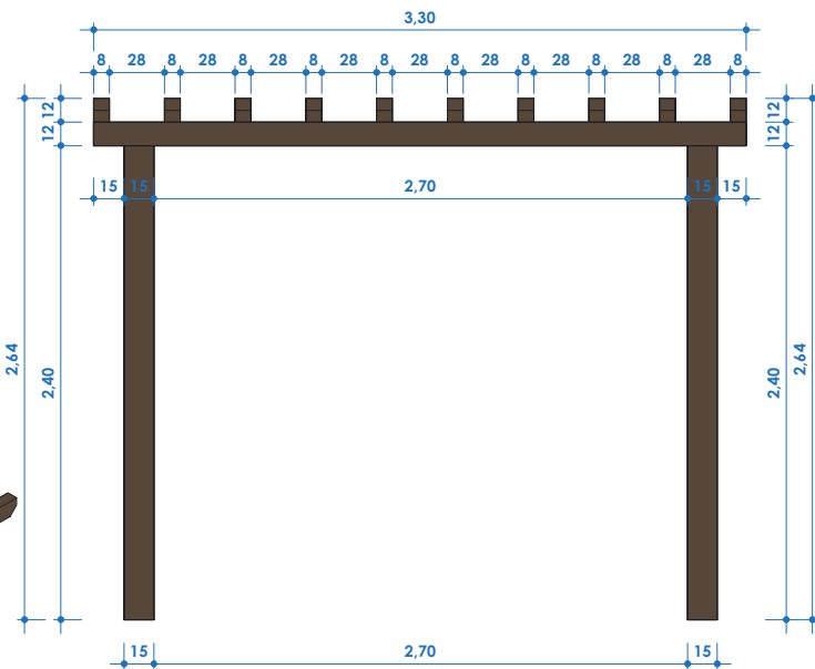
Elevação frontal ESC:1 : 35
